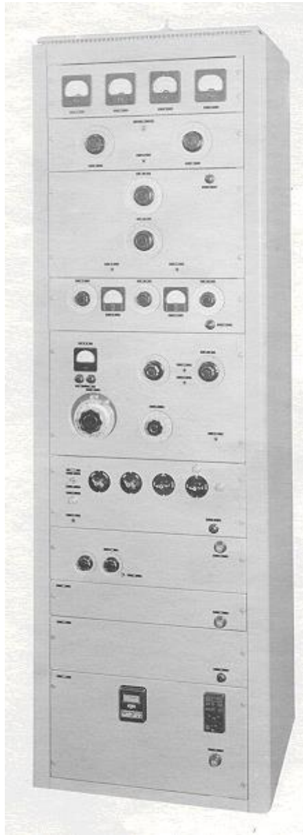
Der Brown Boveri, 300 Watt Kurzwellensender SK 23A, Frequenzbereich: 2.5-24 MHz
