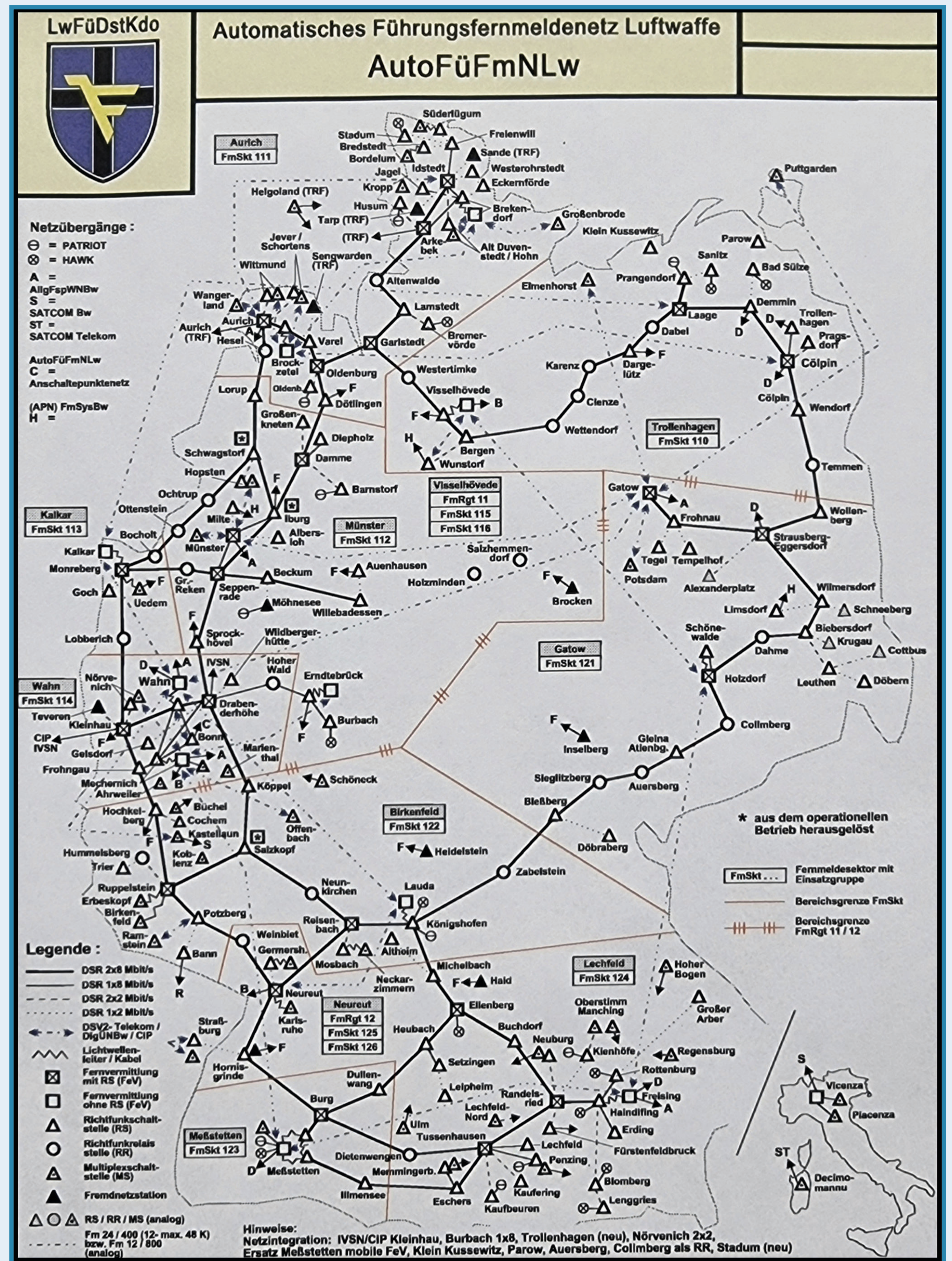
Automatisches Führungs-Fernmeldenetz der Luftwaffe (AutoFüFmNLw)
